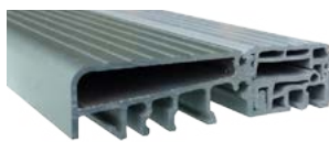
Teplý prah s izoláciou termickou PVC/hliník
